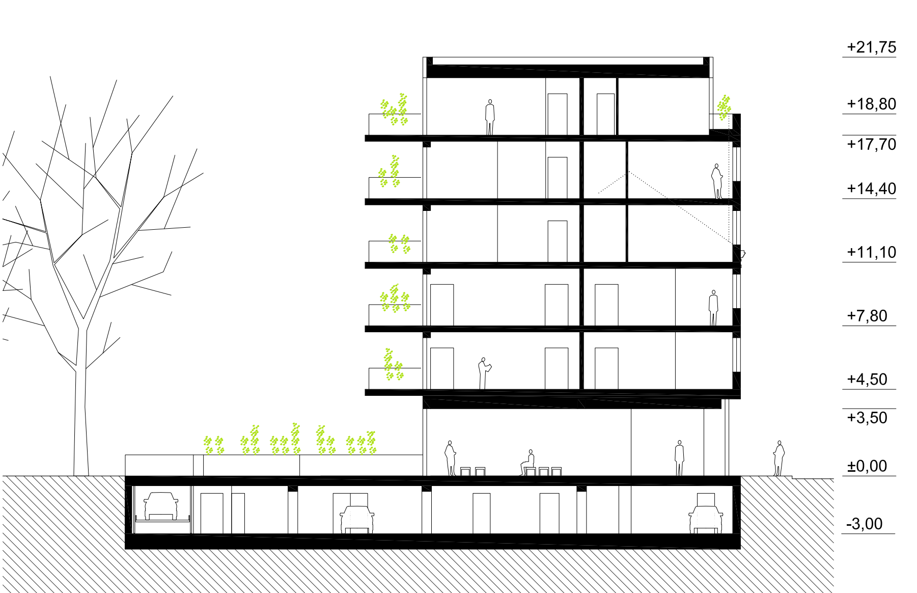
PRESJEK 1-1 M 1:200
